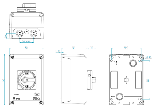
Size EC
